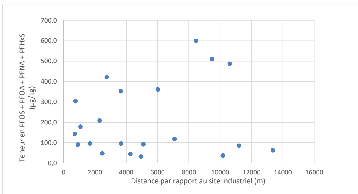
Figure 3. Teneur en PFOS + PFOA + PFNA + PFHxS dans les légumes ( \mu\text{g}/\text{kg} ) en fonction de la distance par rapport au site industriel (m)
